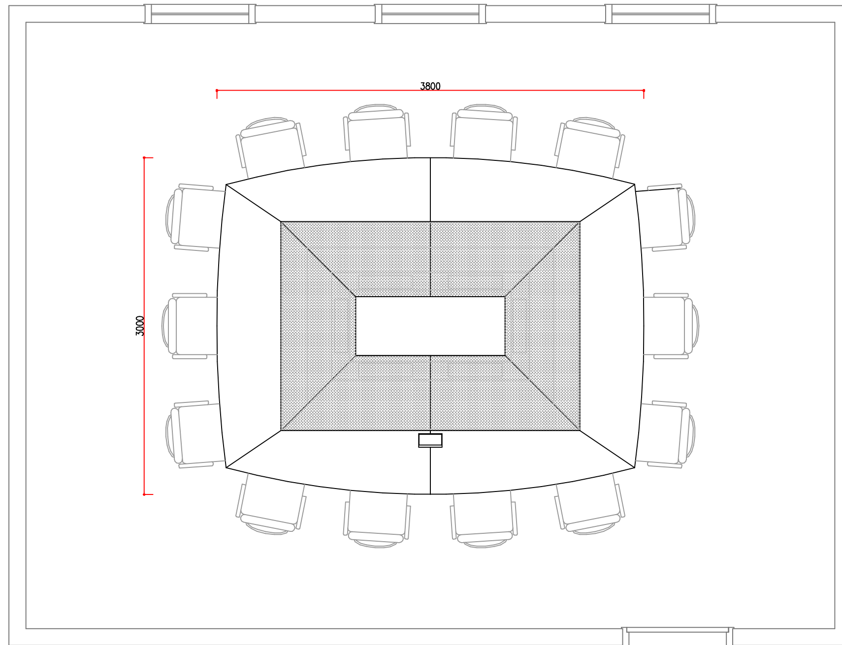
Ruimte 7,20 x 5,40 m1 / Tafel 14-persoons
